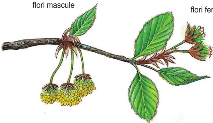
flori masculine
